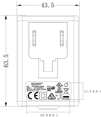
镭雕示意图
