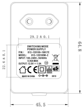
镭雕示意图
